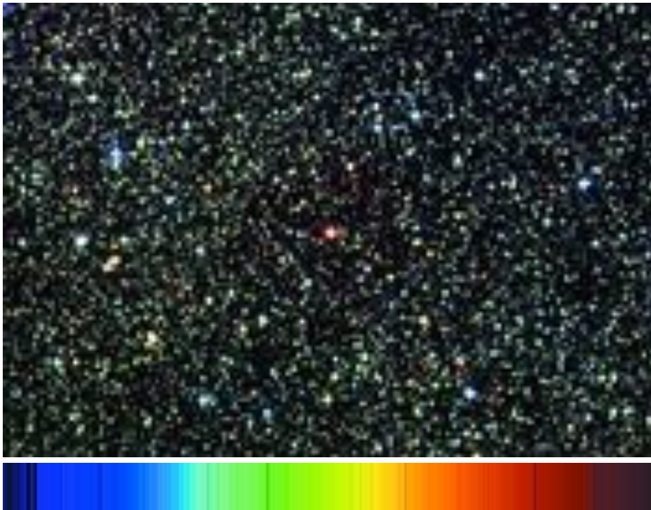
Proxima Centauri, en rød dværgstjerne. Solens spektrum
